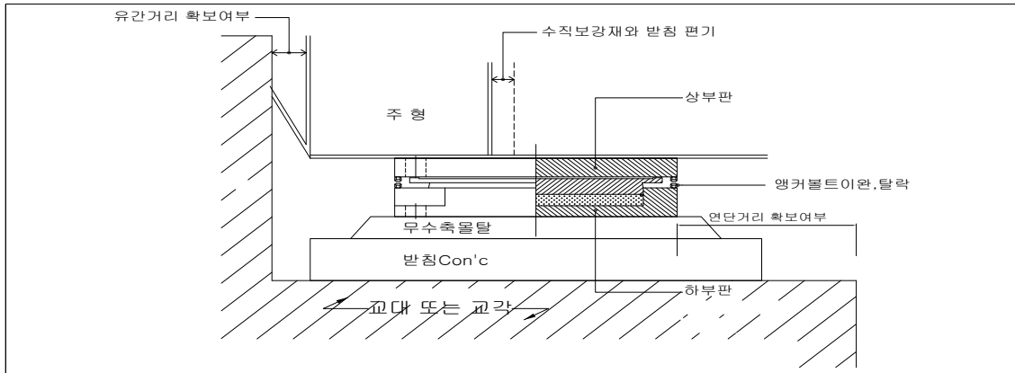
【그림 3.2.15】 교량받침 점검부위
